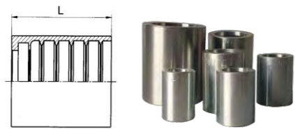
Non-Skive ferrule for 1SN/R1AT-00110
