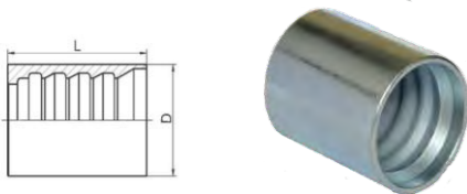
Skive Ferrule for 1SN/R1AT -00100
